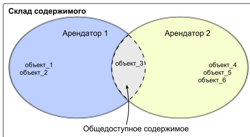
Рисунок 9. Хранилище содержимого, сконфигурированное для использования функций поддержки нескольких арендаторов Cognos BI.
